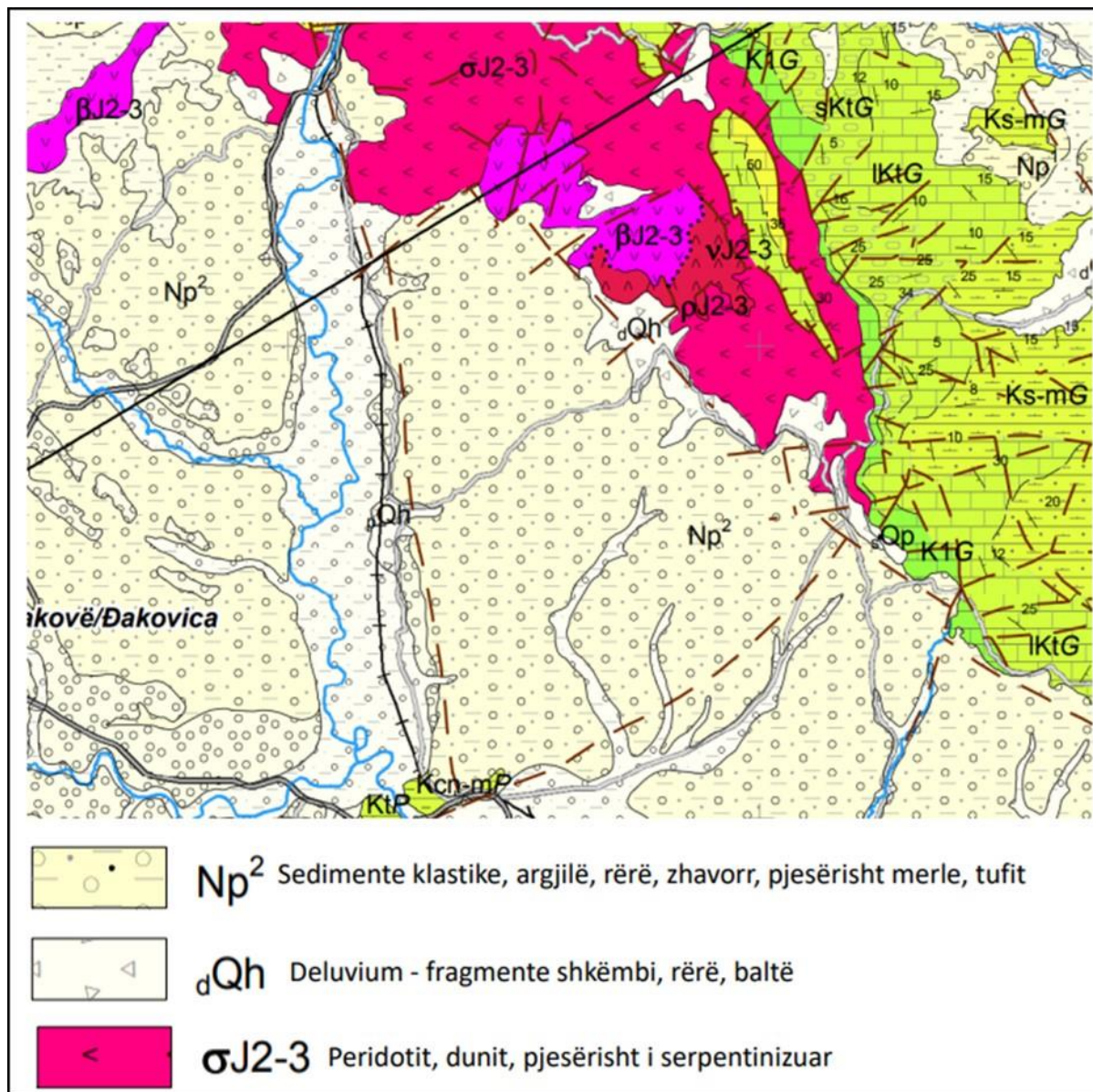
Figura 16. Gjeologjia e zonës ku do të ndërtohet parku solar në Rahovec
