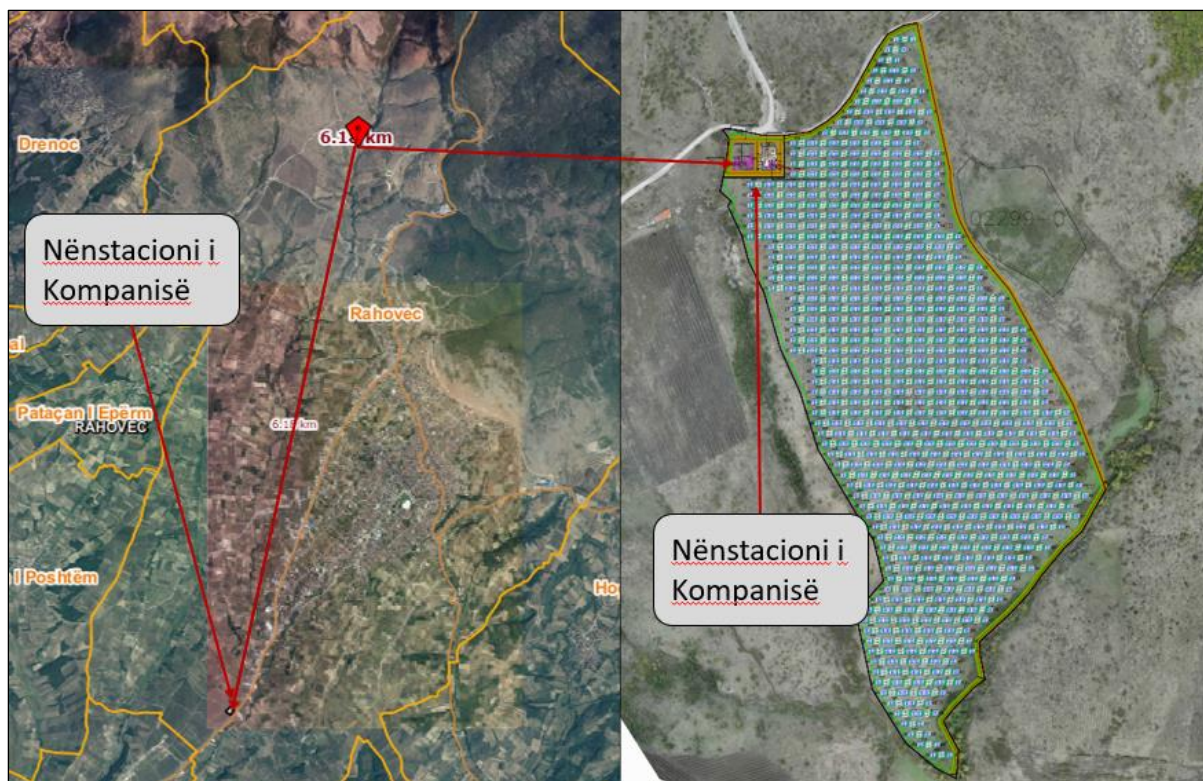
Figura 10 Nënstacioni i kompanisë dhe distanca nga nënstacioni i qytetit
